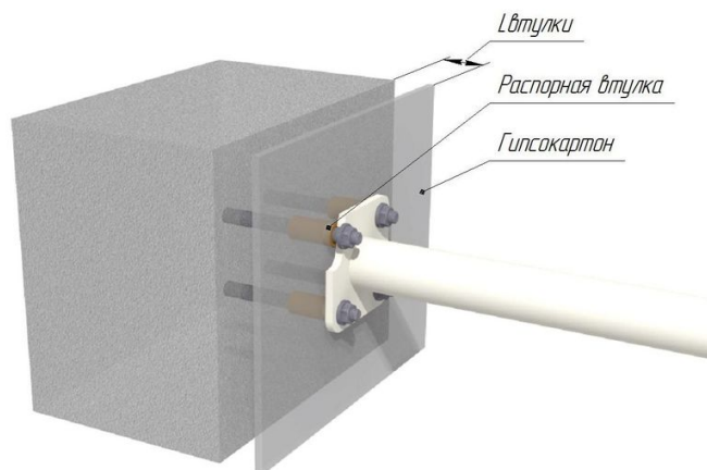
Рис.1. Установка штанги для одежды на стену из гипсокартона
