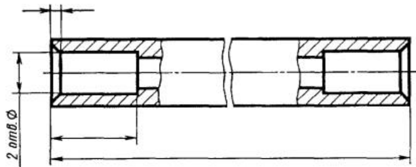
Чертежи деталей
