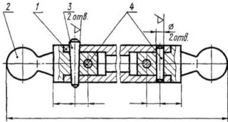
Чертежи деталей
