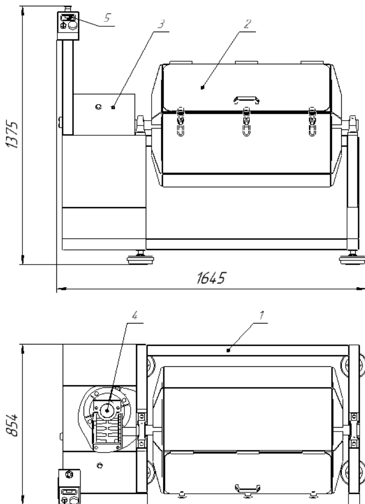
Рис. 1 Схема барабанной галтовки:
