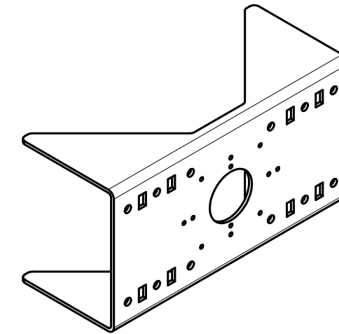
Изометрия 1:4
